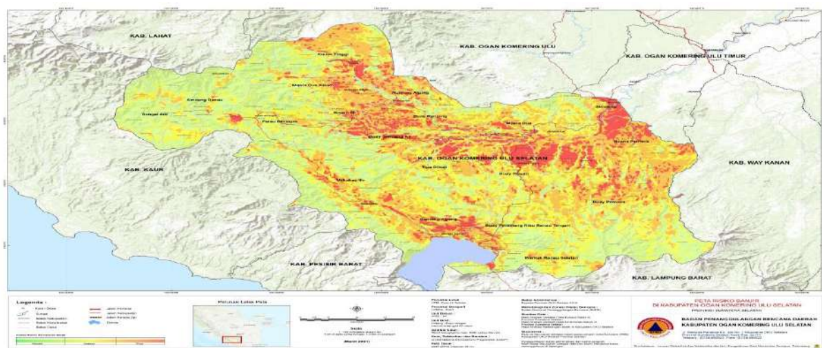
Gambar II. 10 Peta Indeks Resiko Bencana Banjir
