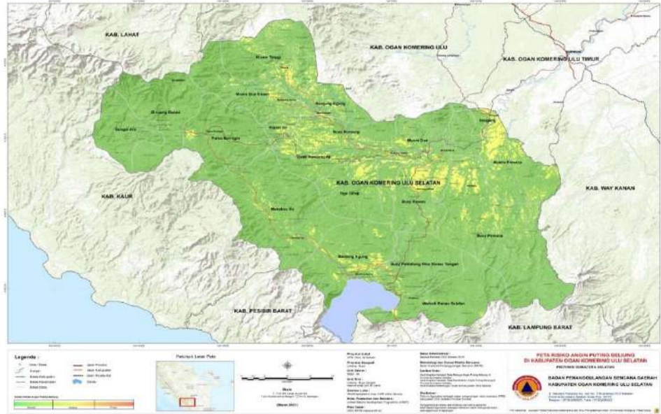
Gambar II. 11 Kawasan Rawan Puting Beliung
