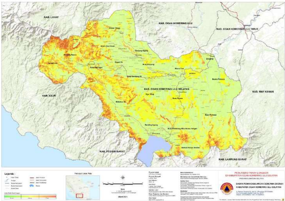
Gambar II. 7 Perkiraan Wilayah Berpotensi Terjadi di Kabupaten OKU SeLatan
